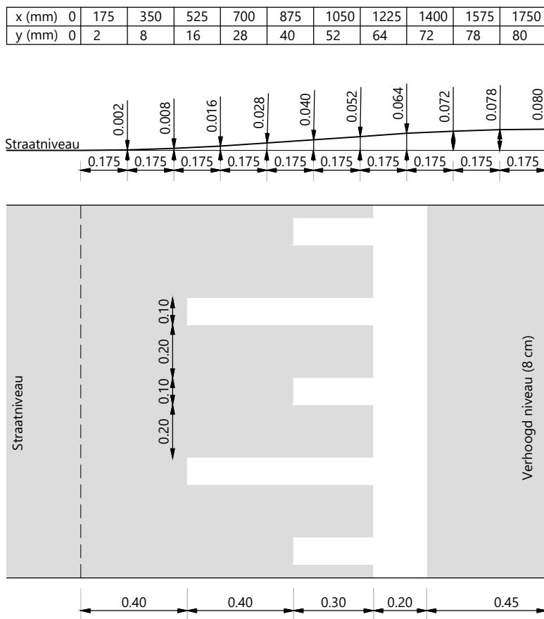
PRINCIPE PROFIEL SINUSDREMPELS 8 cm 30 km/u Schaal 1:20
