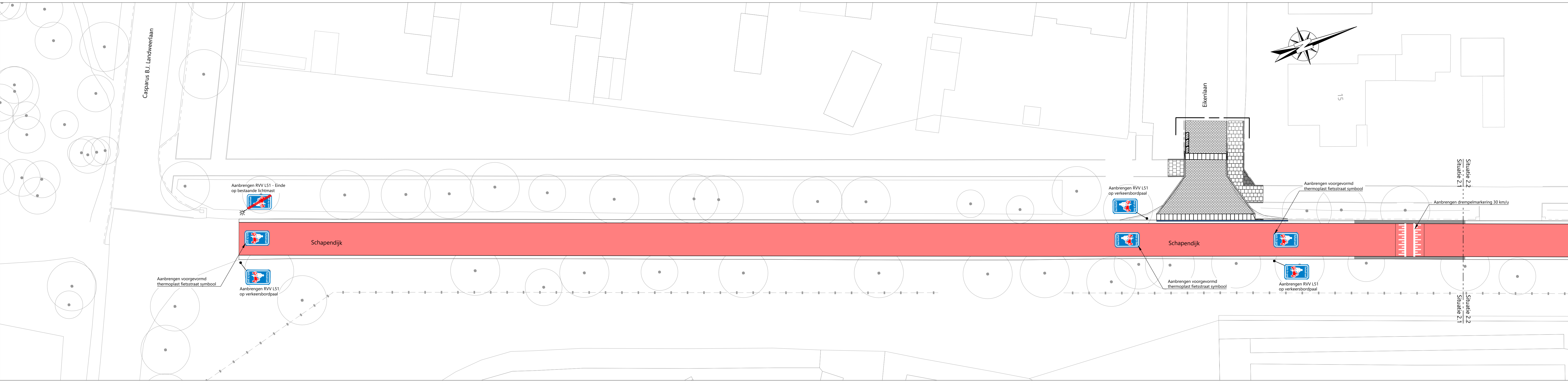
Situatie 2.1 Schaal 1:200
