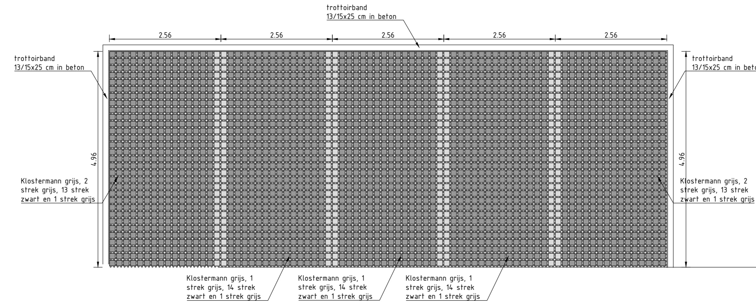
Detail haaksparkeren schaal 1:50
